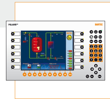
Touch Panel con tecnologia LED
